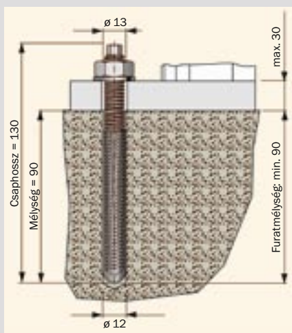
Ragasztópatronos horgonycsavar
