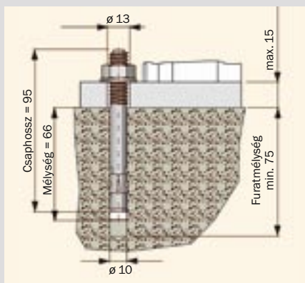
Feszítő horgonycsavar
