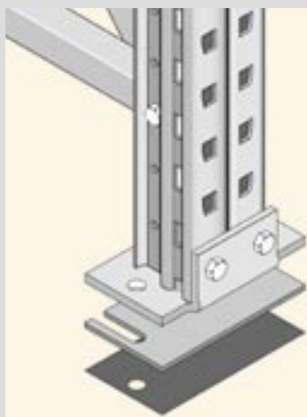
P 73 és P 93 állványláb
