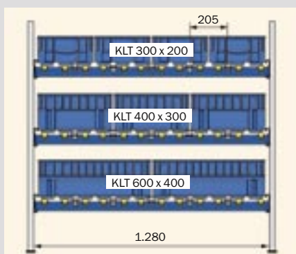
Tiszta mezőszélesség 1.280 mm
