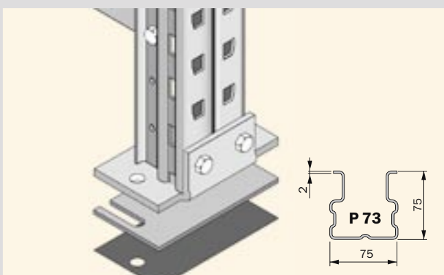
P 73 állványláb
