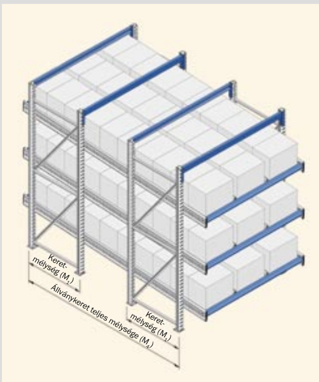
Állványkeretek egymás mögött nagy mélységű tálcához
