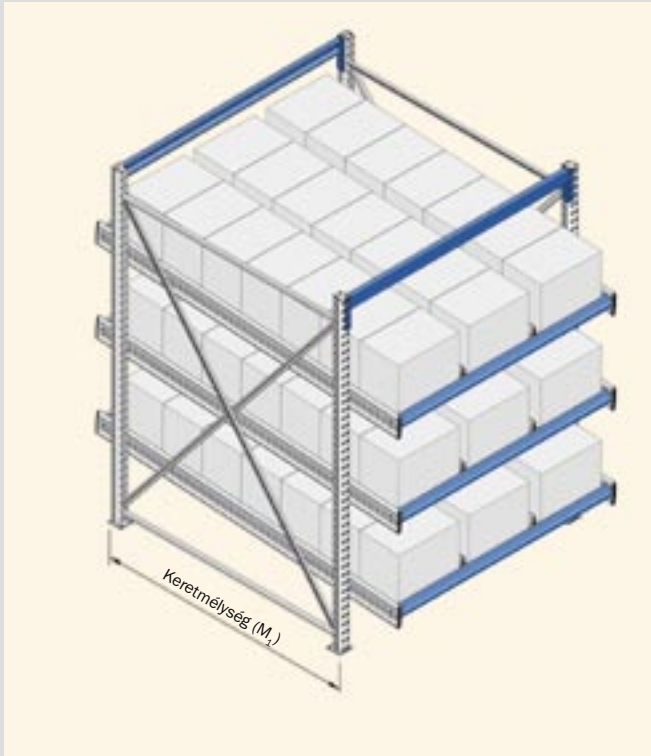
Standard keret (ld. 7. oldal)
