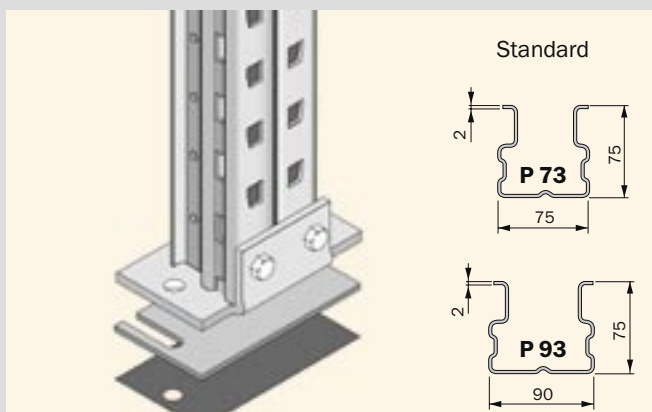
P 73 és P 93 állványláb
