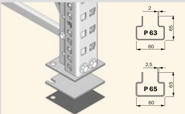
P 63 és P 65 állványláb
