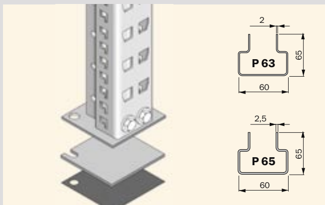
P 63 és P 65 állványláb
