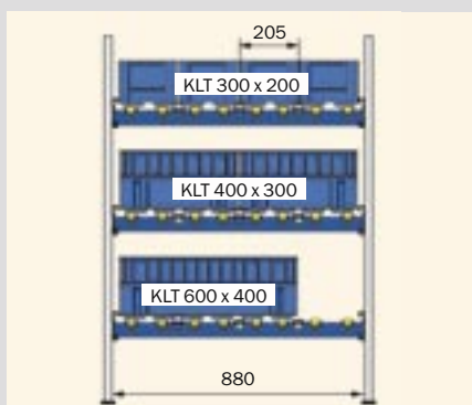
Tiszta mezőszélesség 880 mm
