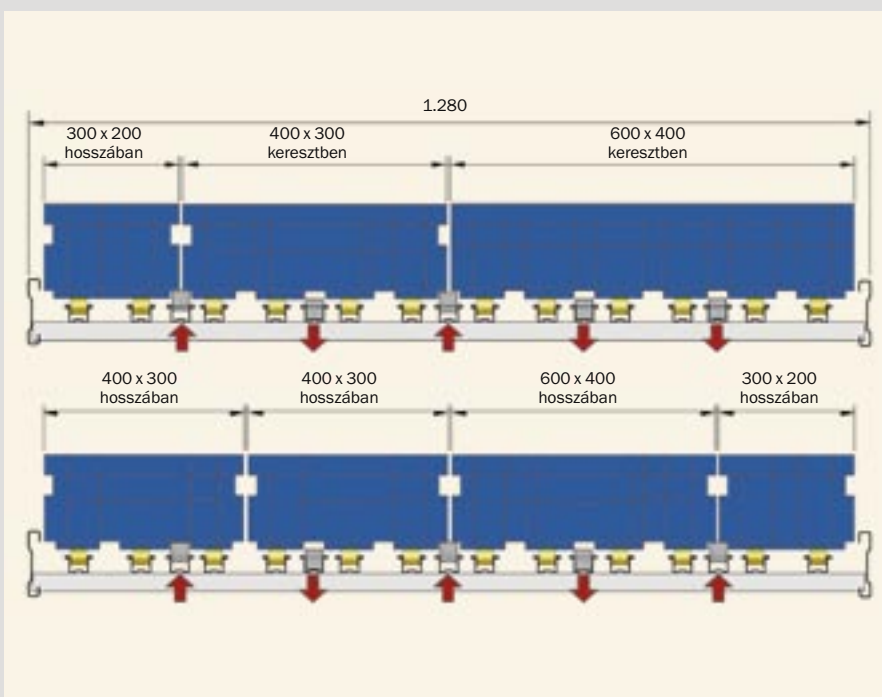
Példa az 1.280 mm-es mezőszélességre
