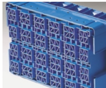
A KLT-doboz stabil fenékbordázata
